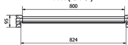
A-A (1 : 8)
