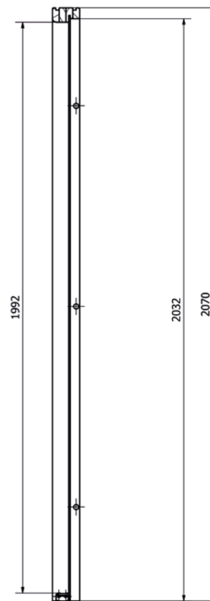
B-B (1 : 8)
